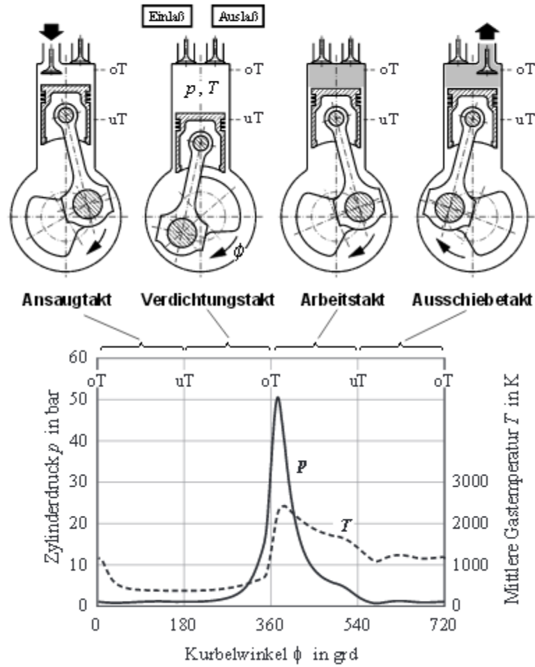
Bild 1: Viertakt-Arbeitsspiel eines Verbrennungsmotors
